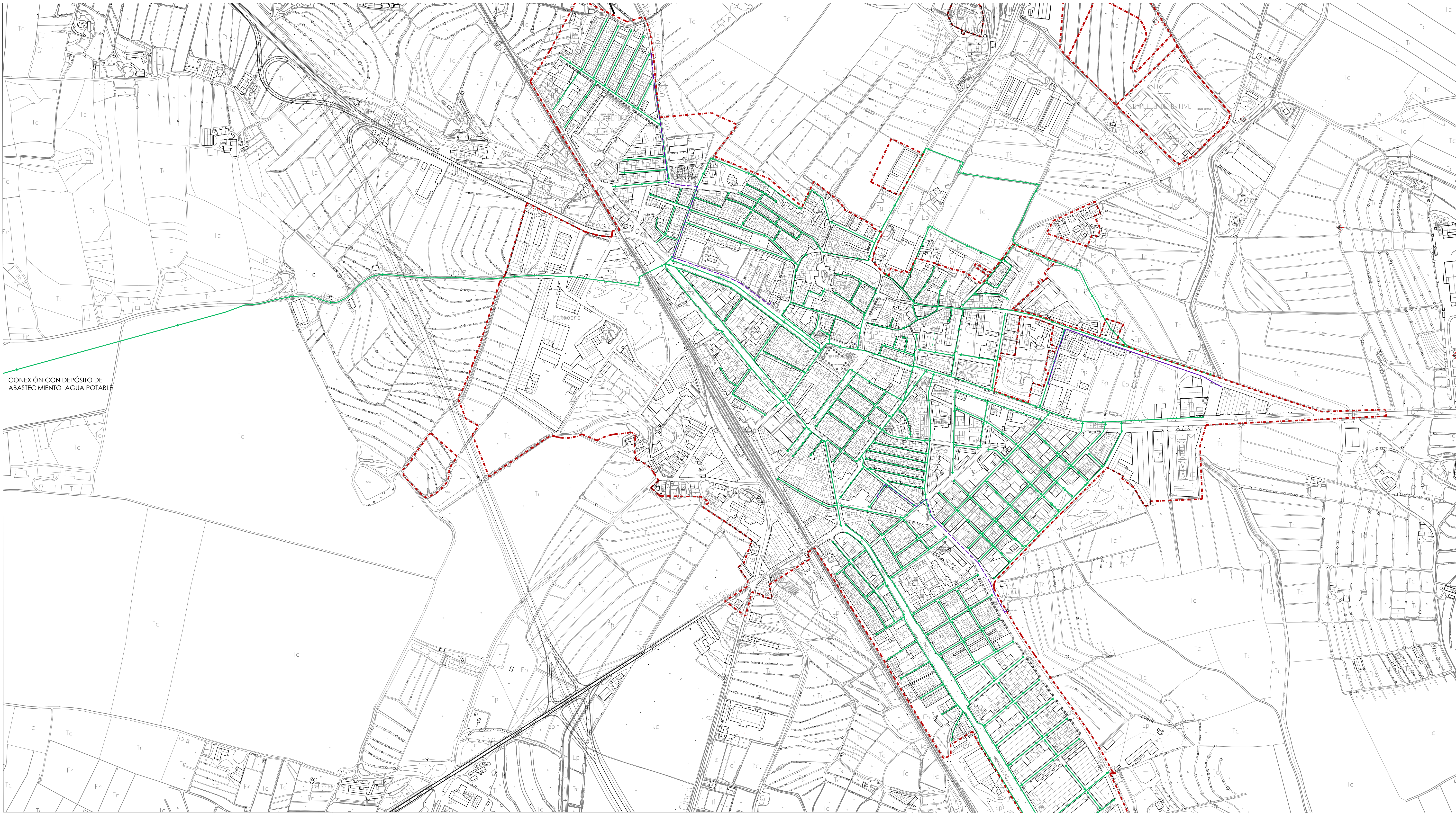
CONEXIÓN CON DEPÓSITO DE ABASTECIMIENTO AGUA POTABLE ESCALA 1 / 5.000
